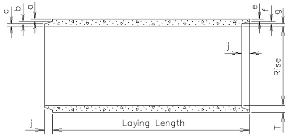
LONGITUDINAL SECTION
